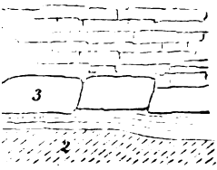
neisskeiles am Gasteinhorn.
